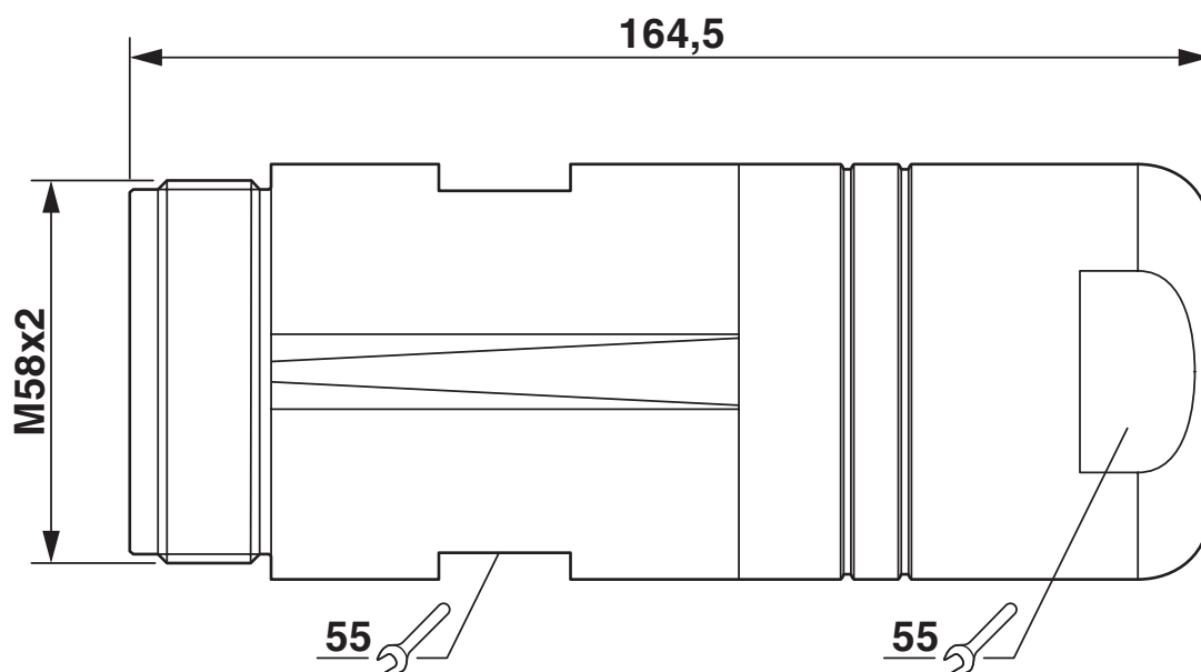
Dessin coté
