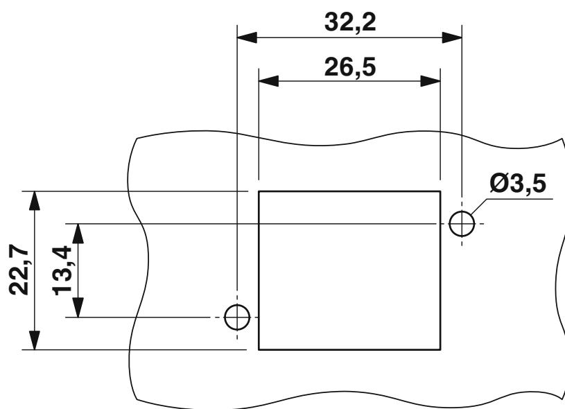
Dessin coté
