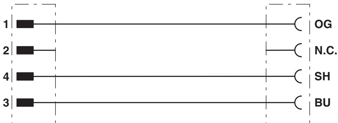
Diagrama eléctrico
