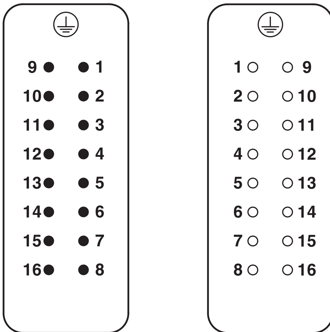
Plano esquemático
