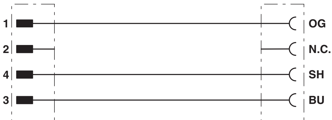
Diagrama eléctrico
