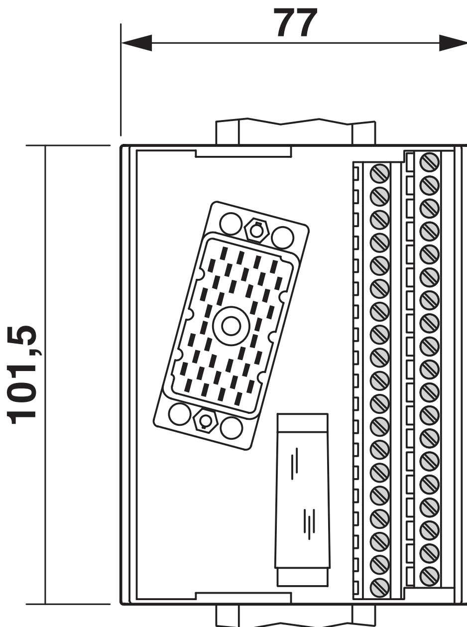
Maßzeichnung
