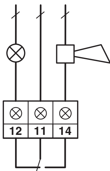
Conexión del contacto de indicación remota en la protección contra sobretensiones
