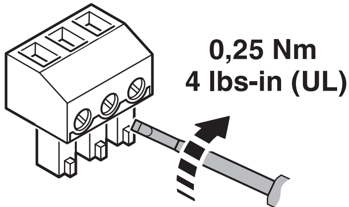
Raccordement du contact de signalisation à distance au niveau de la protection antisurtension
