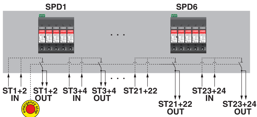
Schéma de l'application schématique
