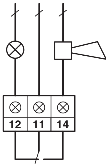
Raccordement du contact de signalisation à distance au niveau de la protection antisurtension
