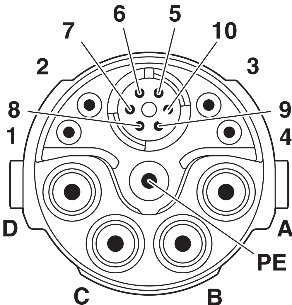
Plano esquemático
