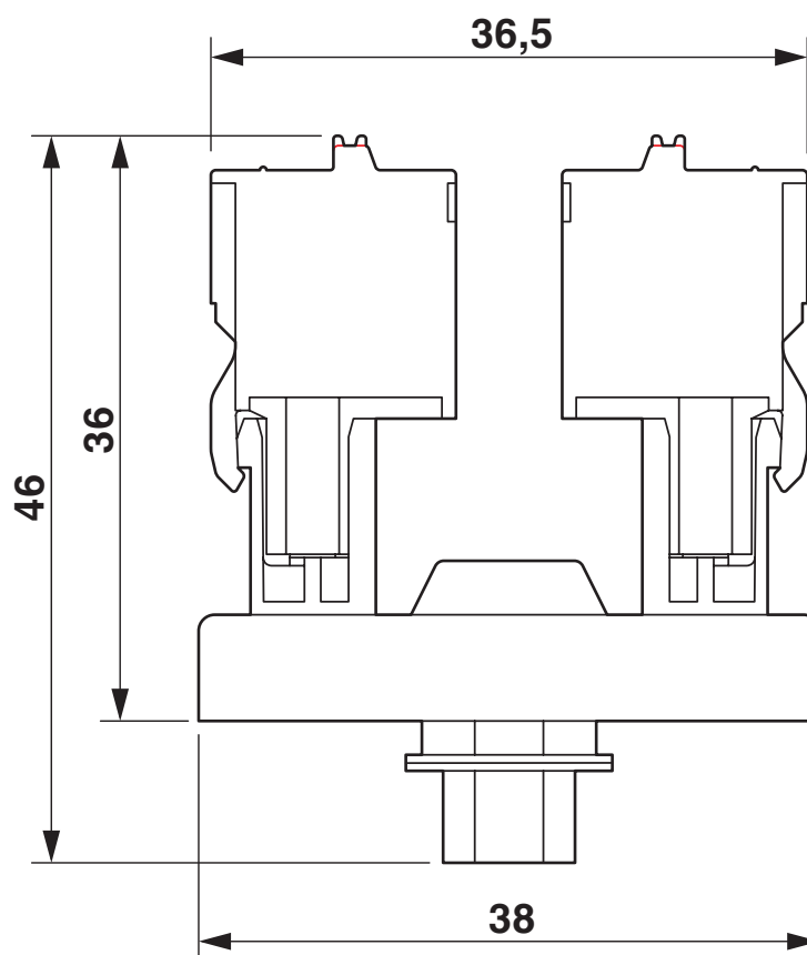
Dessin coté
