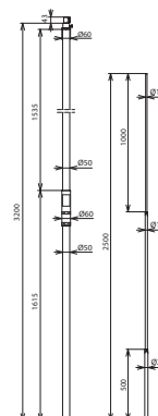
Maßbild SR D50 3200 FS22 2500 IP HVI GFK
