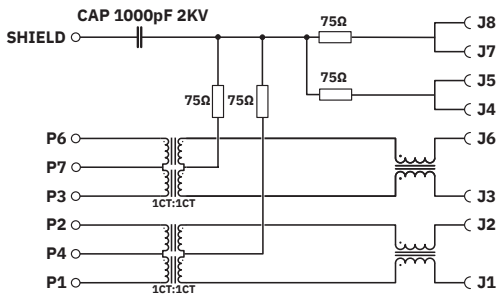
Schaltplan
