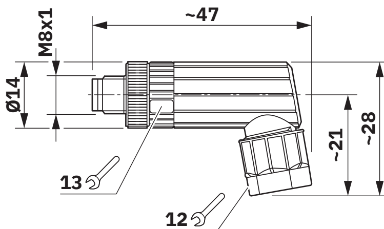
Dessin coté
