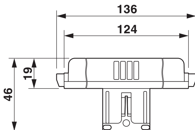
Dessin coté
