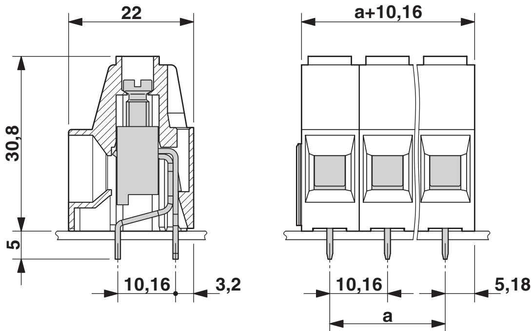
Maßzeichnung
