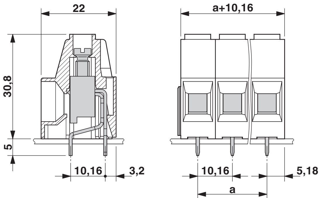
Dessin coté
