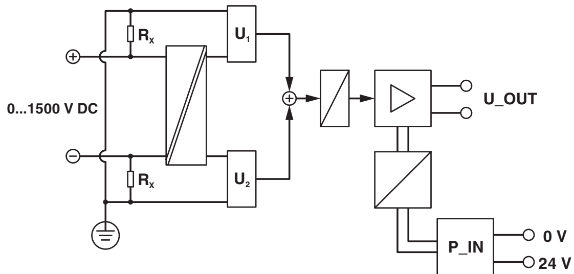
Blockschaltbild
