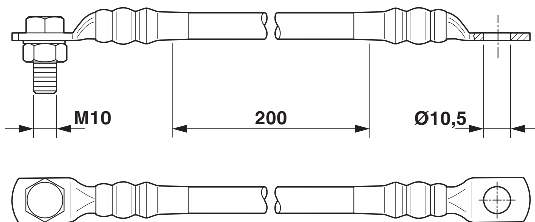
Dessin coté
