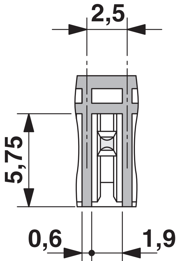
Maßzeichnung
