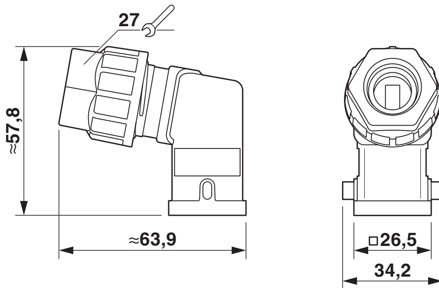
Maßzeichnung
