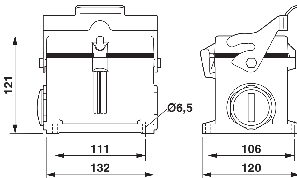
Dessin coté
