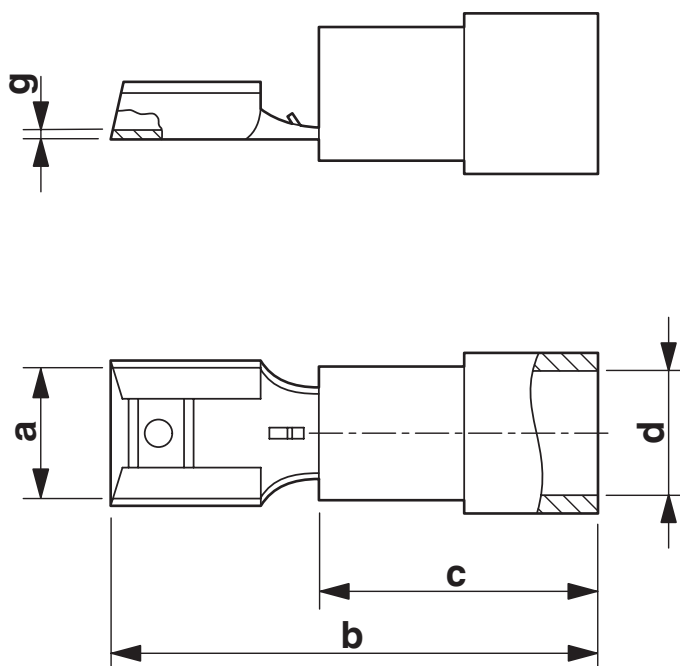
Dessin coté
