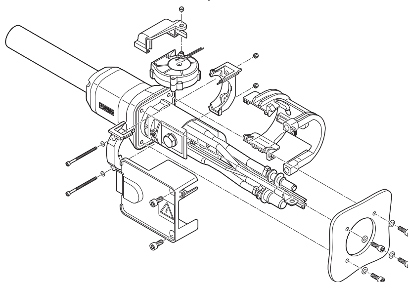
Plano esquemático
