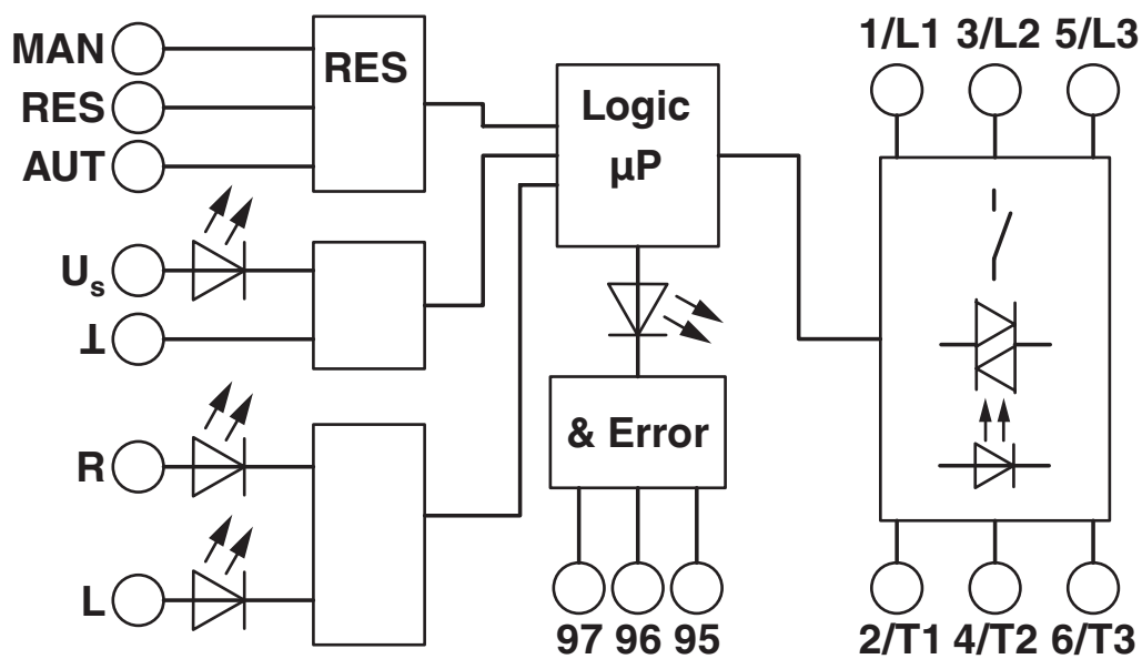
Blockschaltbild
