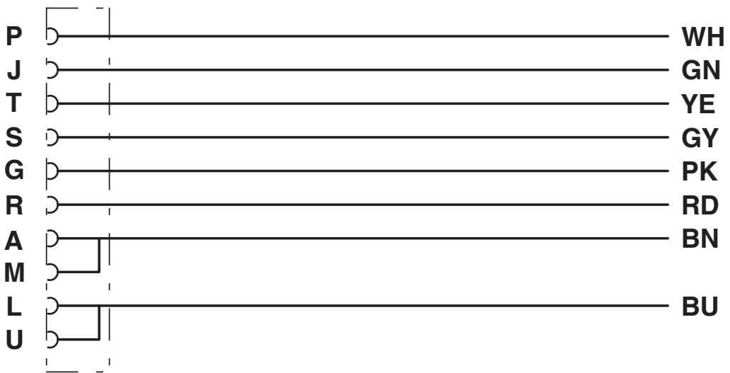
Ocupación de contactos del conector hembra M16
