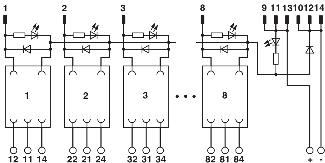
Schaltplan
