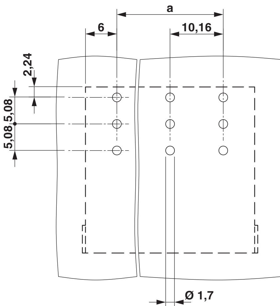
Esquema de taladros/geometría pads soldadura
