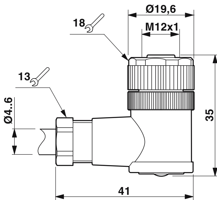
Esquema de dimensiones
