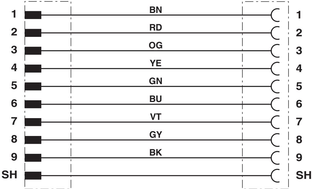
Diagrama eléctrico
