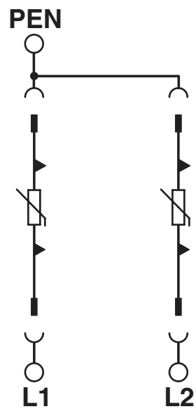
Schaltplan
