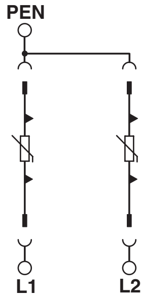
Diagrama eléctrico
