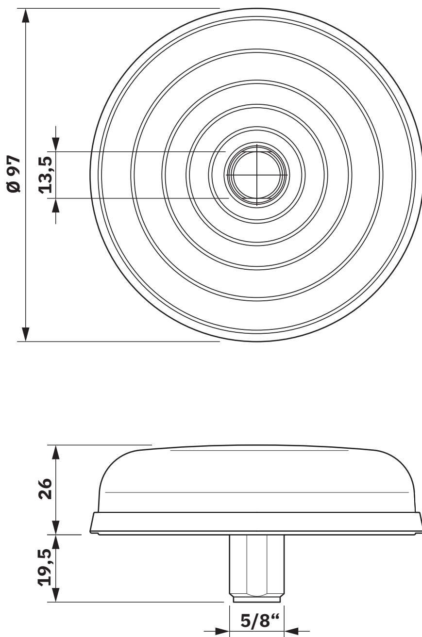
Dessin coté
