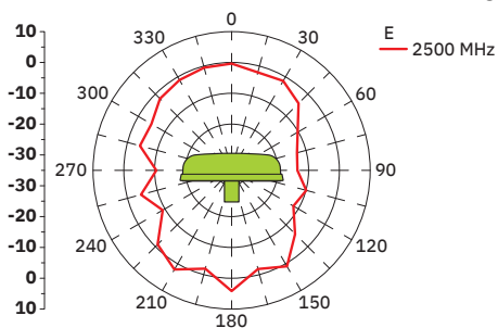
Caractéristiques de rayonnement 2500 MHz
