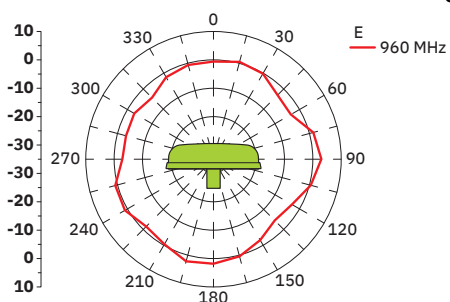
Caractéristiques de rayonnement 960 MHz
