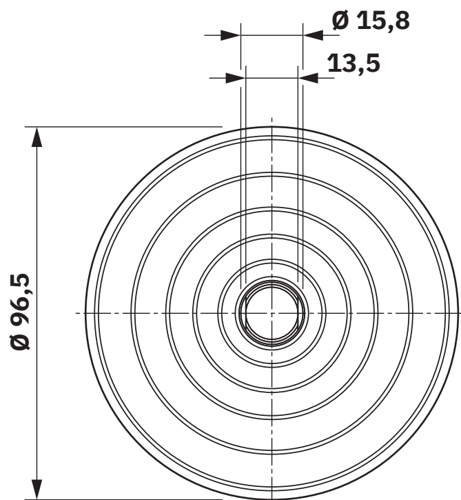
Dessin coté
