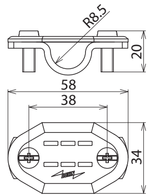
Maßbild NST 16 ON AL
