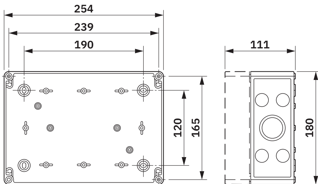
Dimensiones de la carcasa
