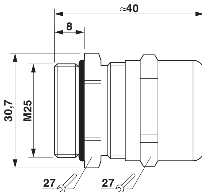
Maßzeichnung
