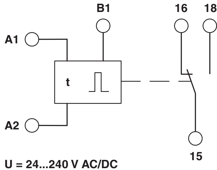
Schéma fonctionnel
