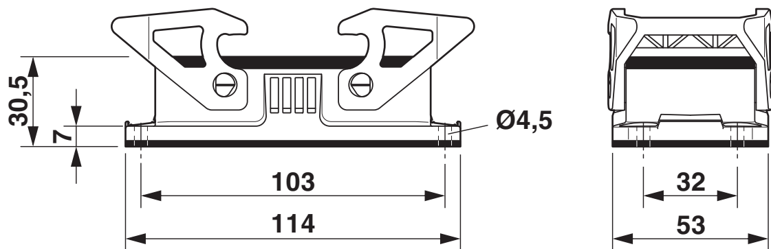
Dessin coté
