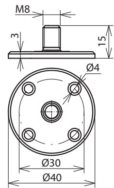
Maßbild BP D40 GBM8 4XB4 K GR
