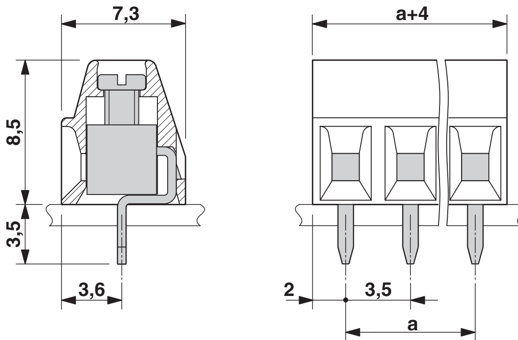
Maßzeichnung
