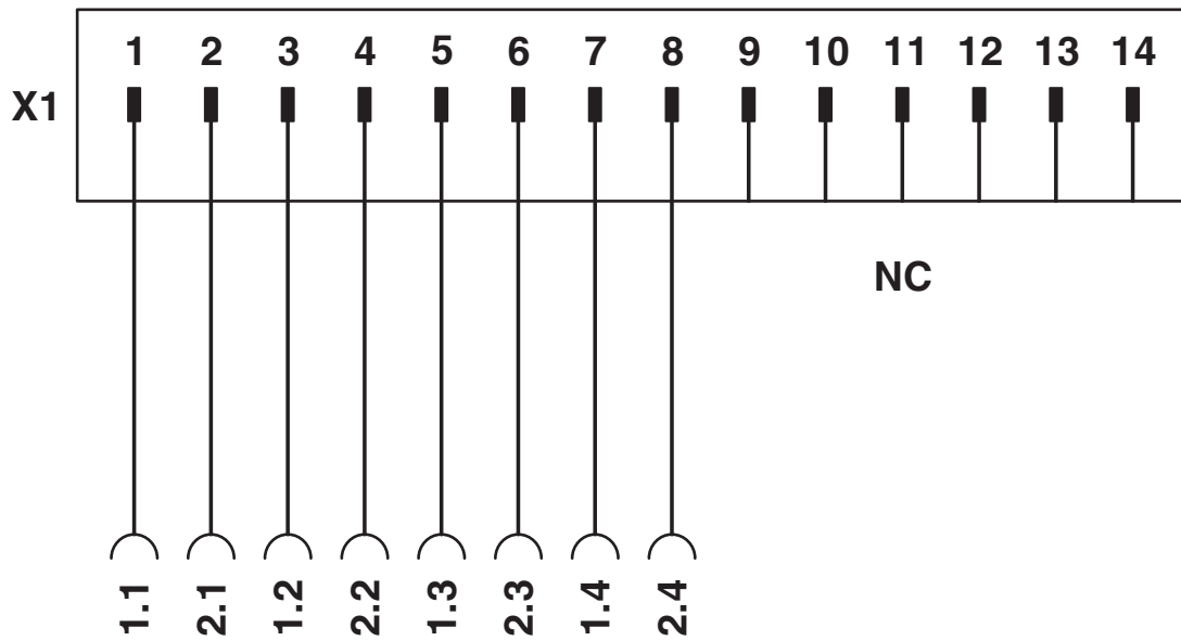
Anschlussbild FLKM 14-PA-INLINE/DIO8
