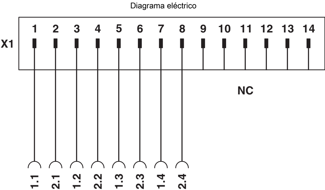
Esquema de conexiones FLKM 14-PA-INLINE/DIO8
