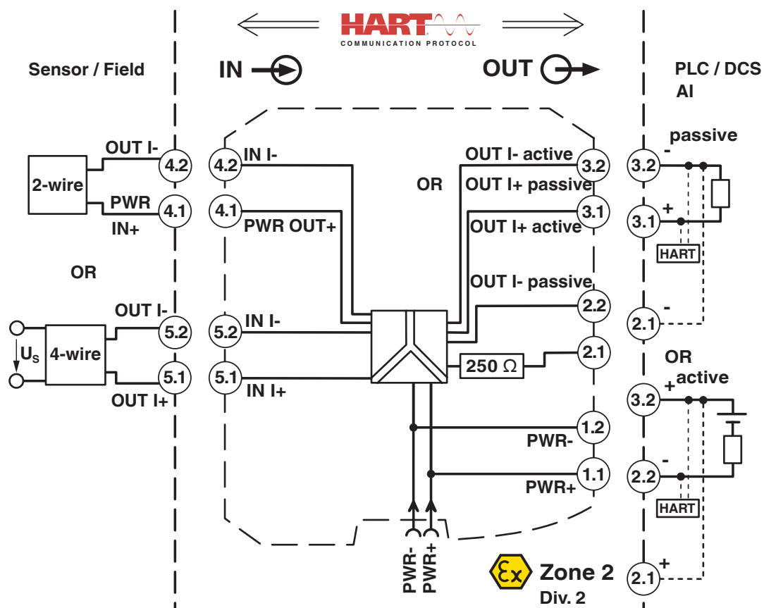
Blockschaltbild
