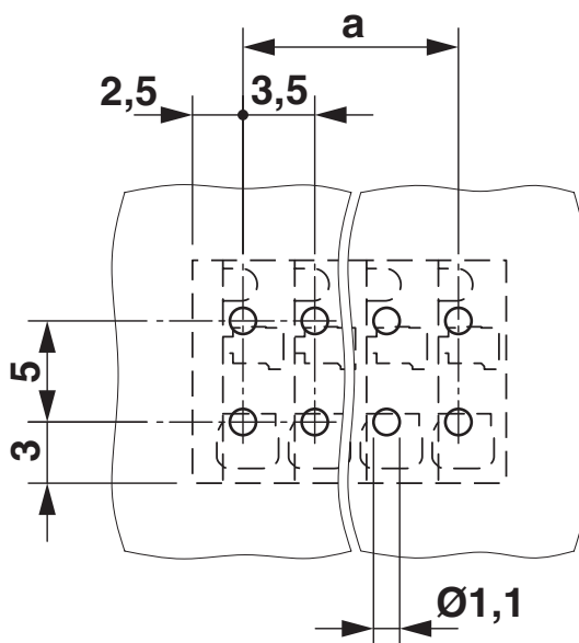
Bohrplan/Lötpadgeometrie
