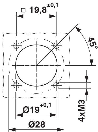
Schemazeichnung
