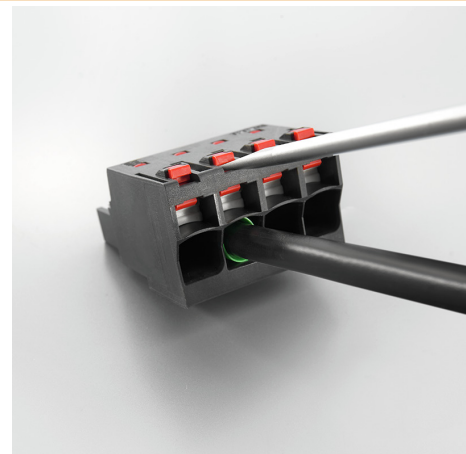
Schnelles Verdrahten
