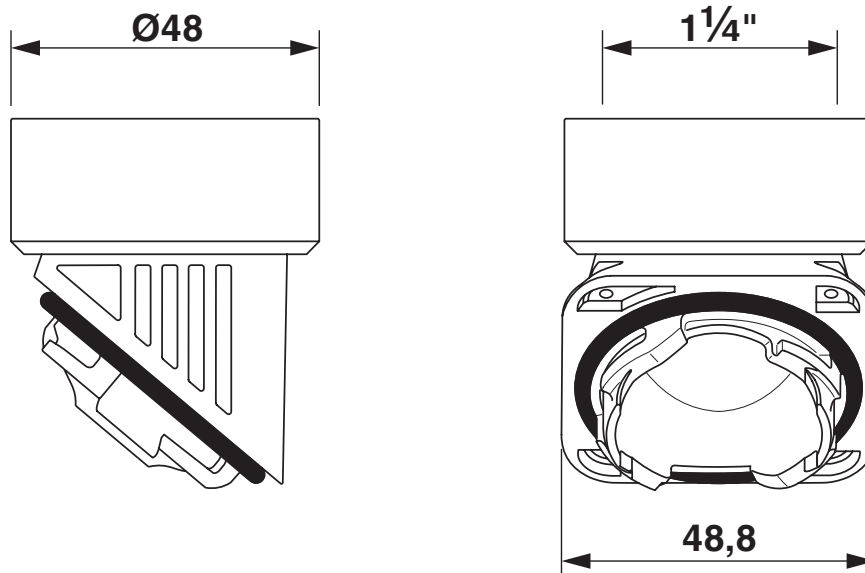
Maßzeichnung
