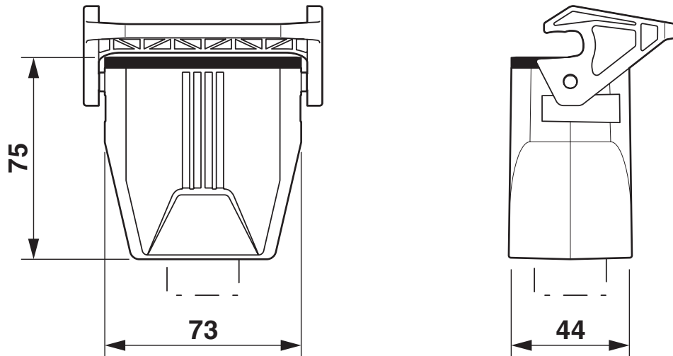
Maßzeichnung
