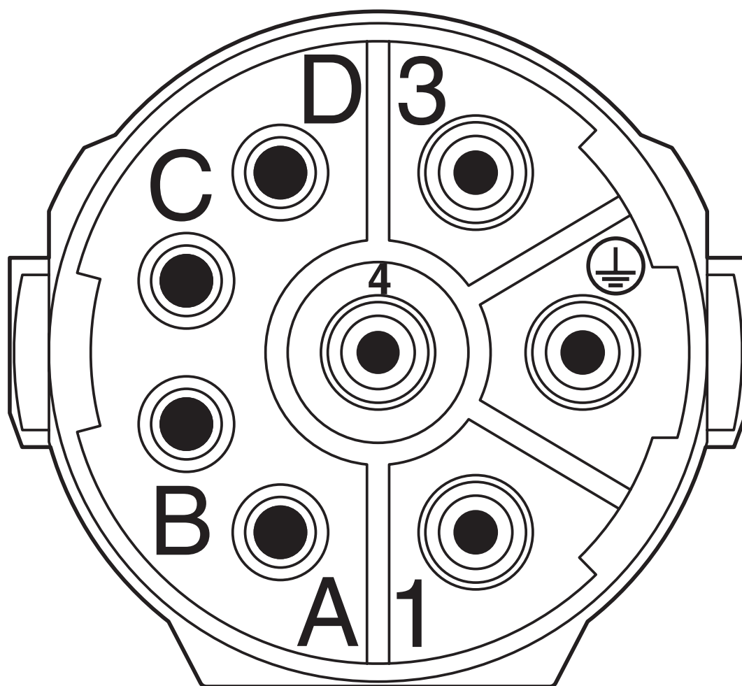
Dessin schématique
