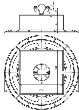
Maßbild DLH ZS 27 V2A BES180 GP300 K
