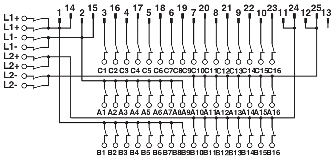
Schéma des connexions FLKM-D25 SUB/B/KDS3-MT/TU830
